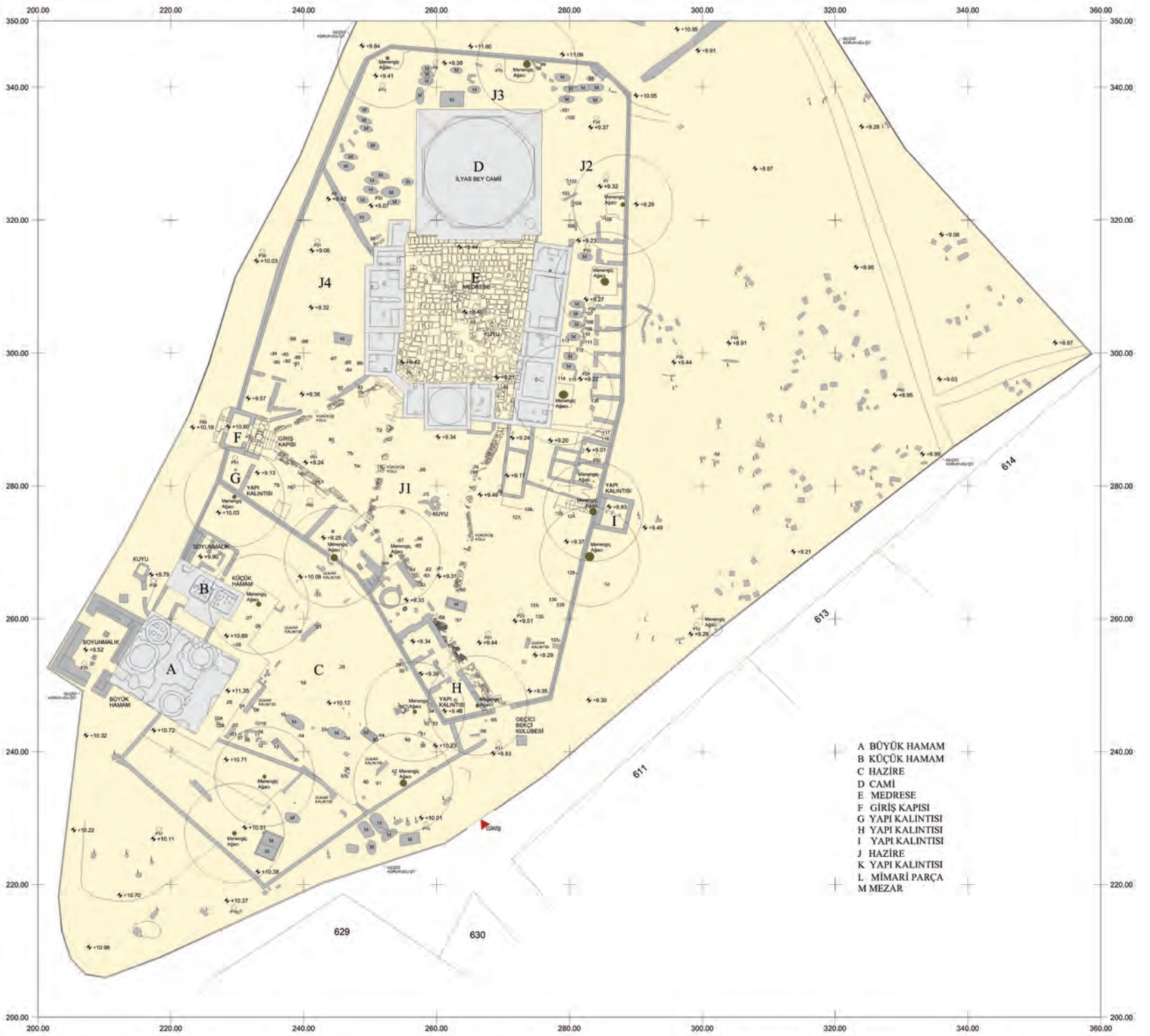
Şekil 1 Balat İlyas Bey Külliyesi. Vaziyet Planı.
